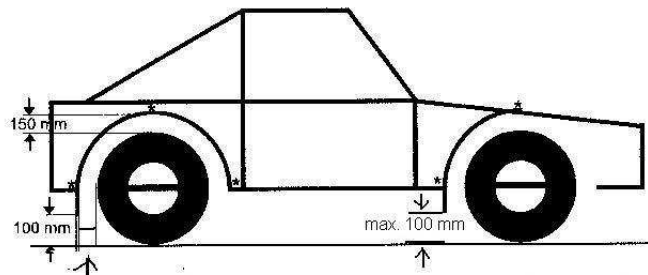
Anbringung Zwischenfahrerschutz
